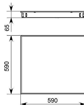
Рисунок 1 – Габаритные размеры светильника
