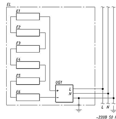
Рисунок 2 – Электрическая схема подключения
