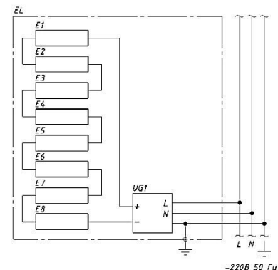
Рисунок 2 – Электрическая схема подключения
