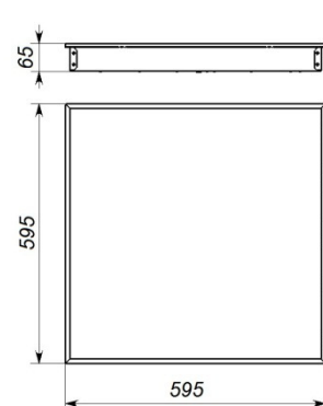
Рисунок 1 – Габаритные размеры светильника
