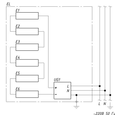
Рисунок 2 – Электрическая схема подключения
