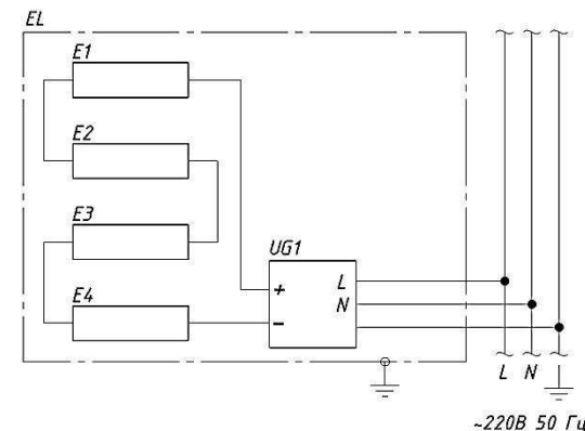
Рисунок 2 – Электрическая схема подключения
