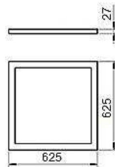
Рисунок 1 – Габаритные размеры светильника
