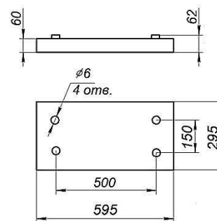
Рисунок 1 – Габаритные размеры светильника
