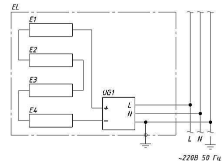
Рисунок 2 – Электрическая схема подключения
