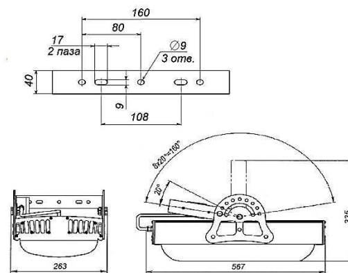
Рисунок 1 – Габаритные размеры прожектора
