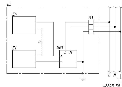
Рисунок 2 – Электрическая схема подключения
