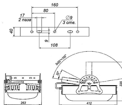
Рисунок 1 – Габаритные размеры прожектора
