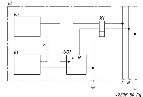
Рисунок 2 – Электрическая схема подключения
